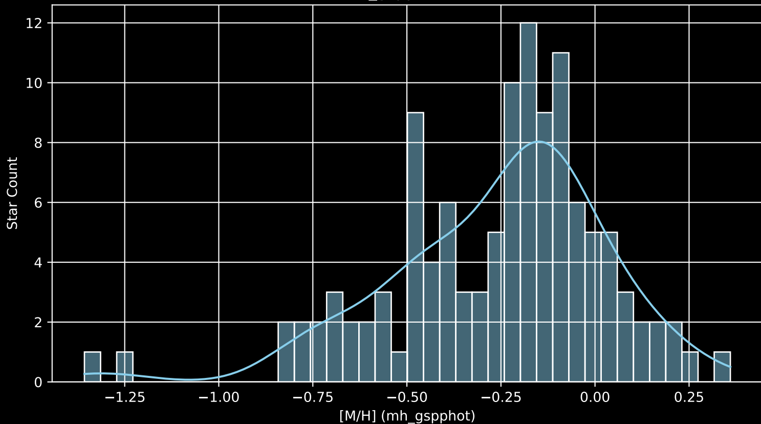
GALAH DR4 Field: [6692] [M/H] (mh_gspphot) (n= 118)
