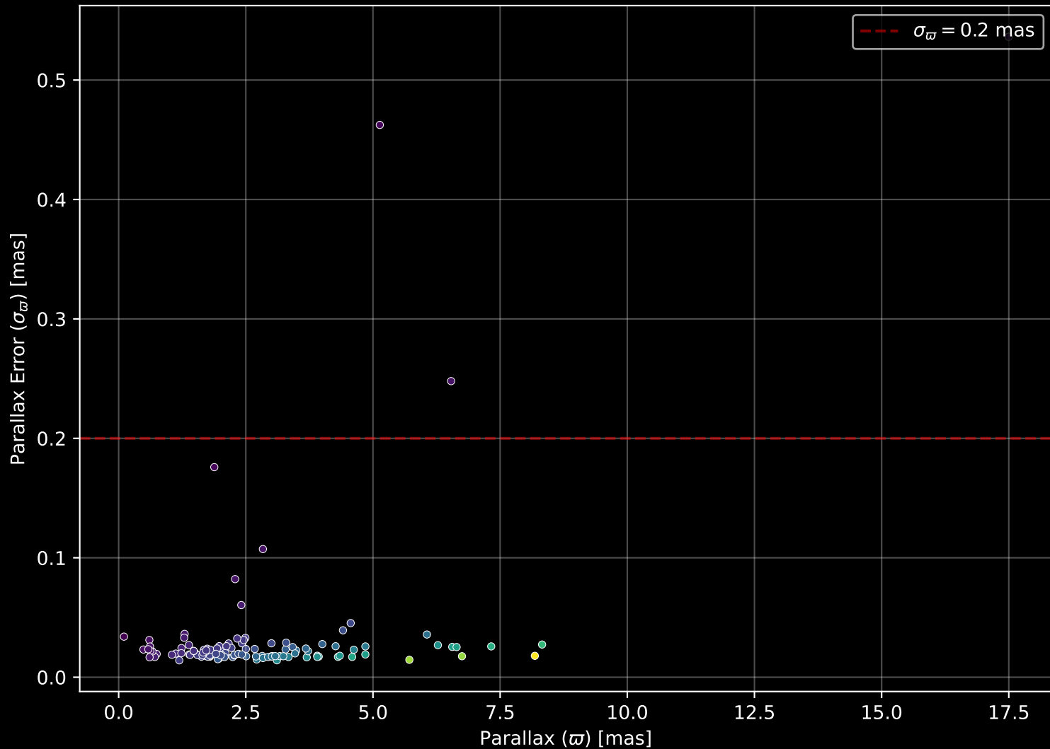
GALAH DR4 Field: [6692] Parallax Quality (n= 118)
