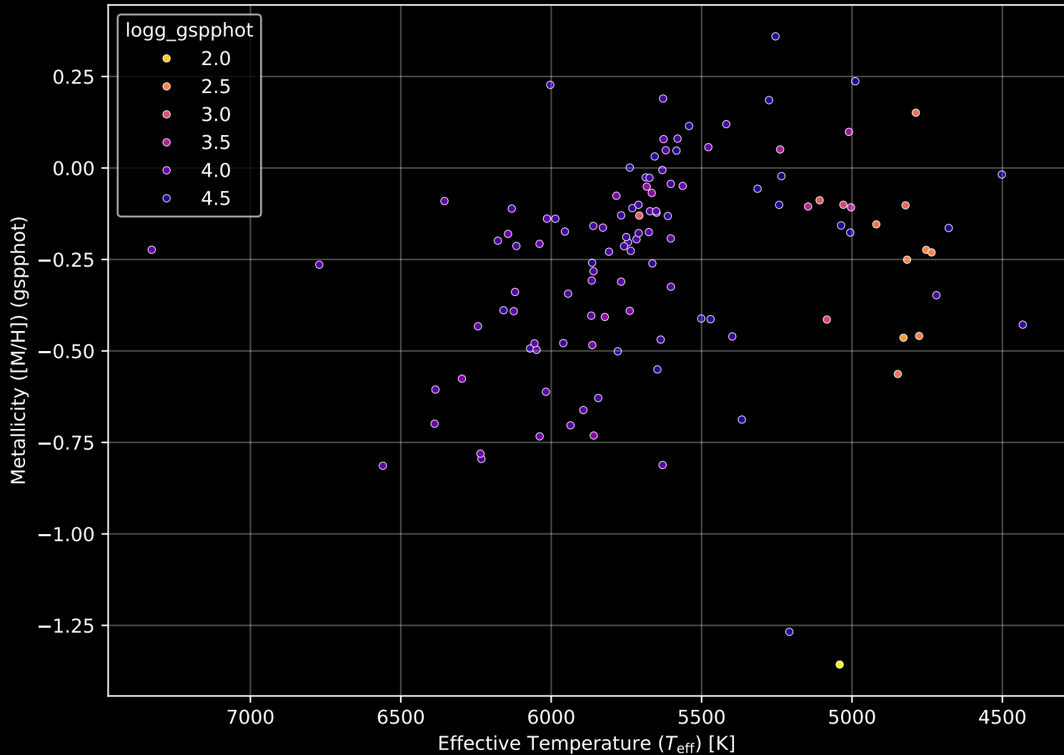
GALAH DR4 Field: [6692] Stellar Population Parameters (n= 118)
